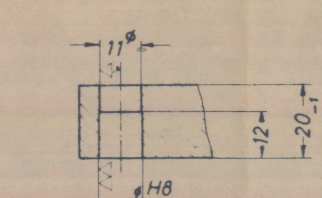
Schnitt C-D
