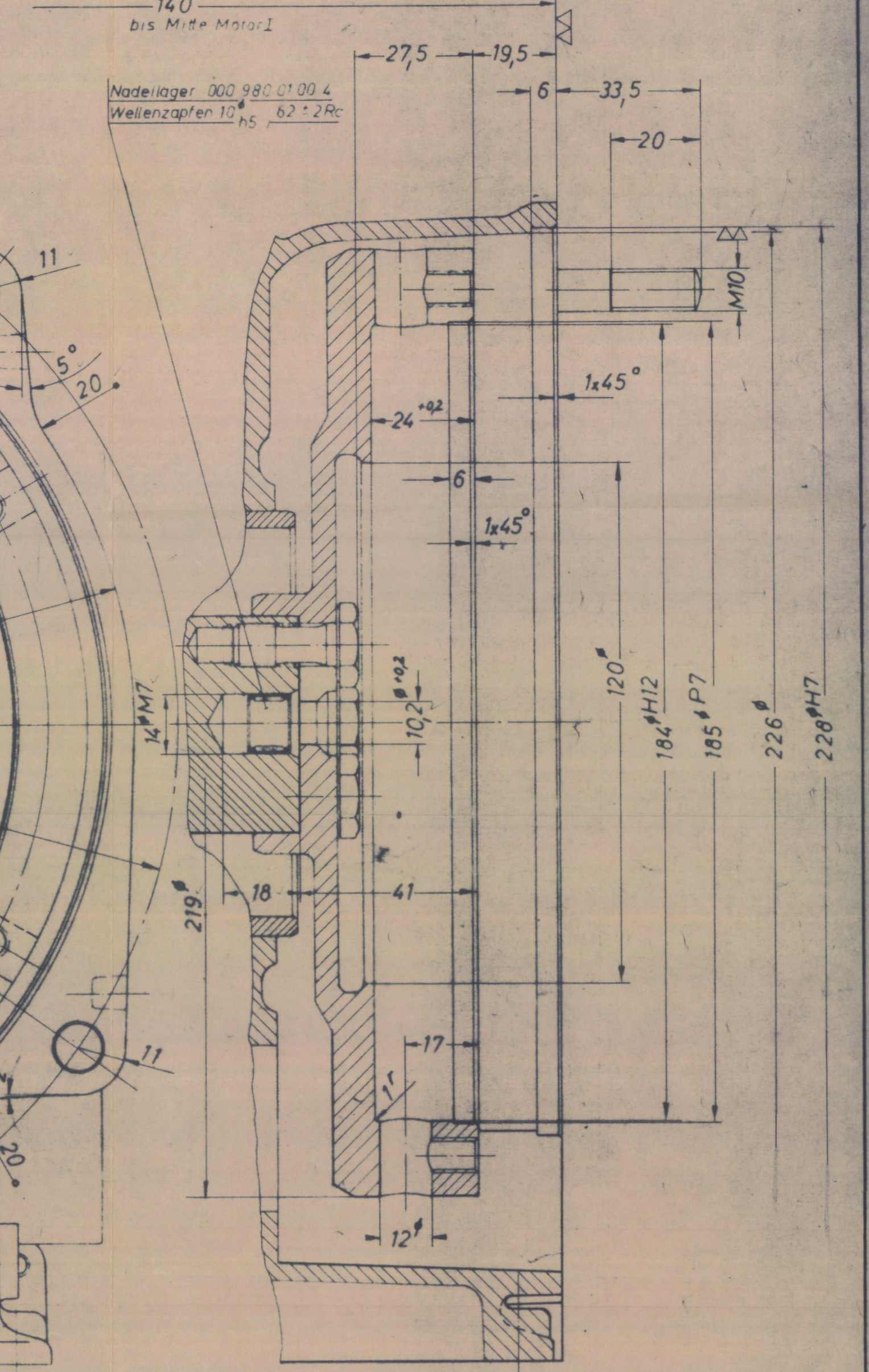
Schnitt A-B
