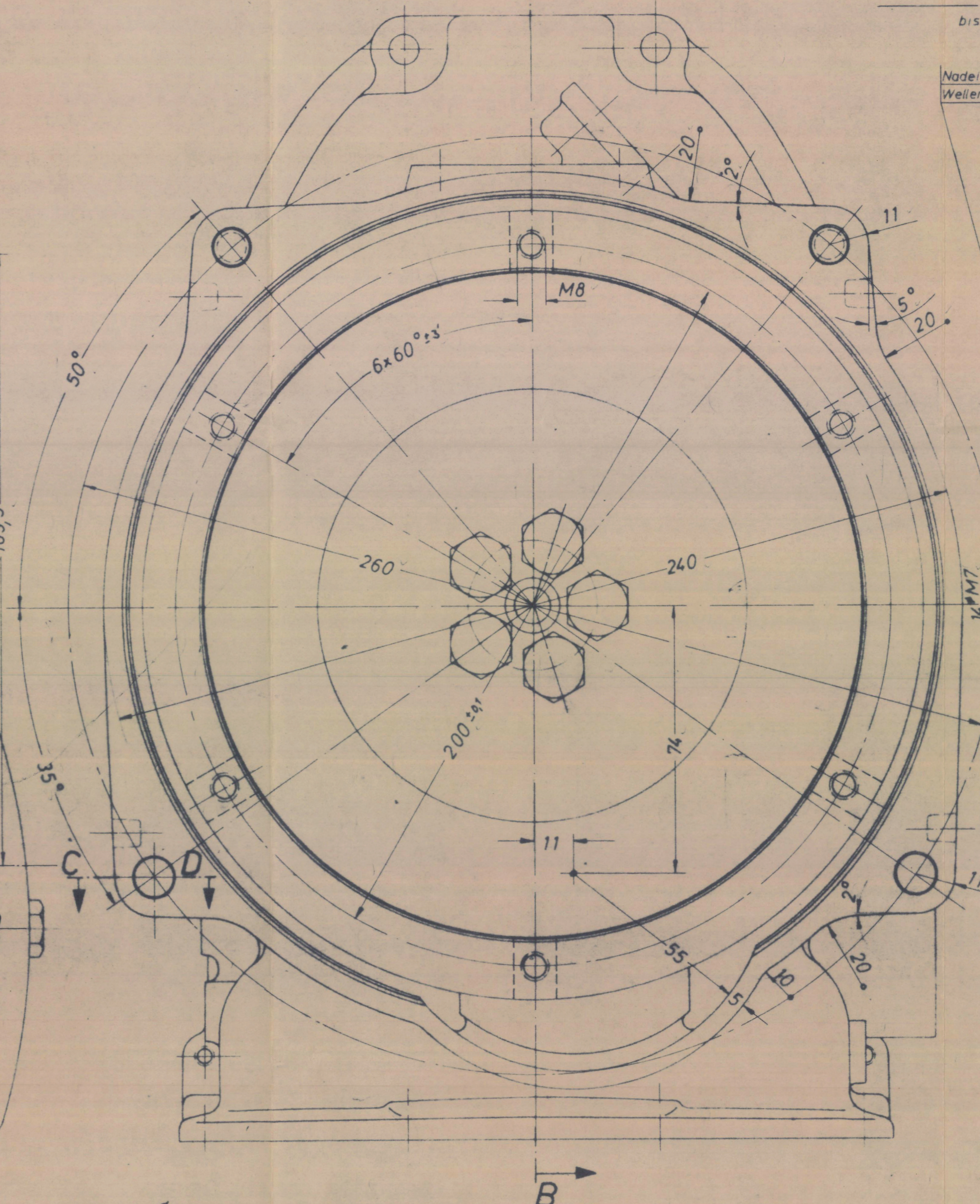
Ansicht „A“
